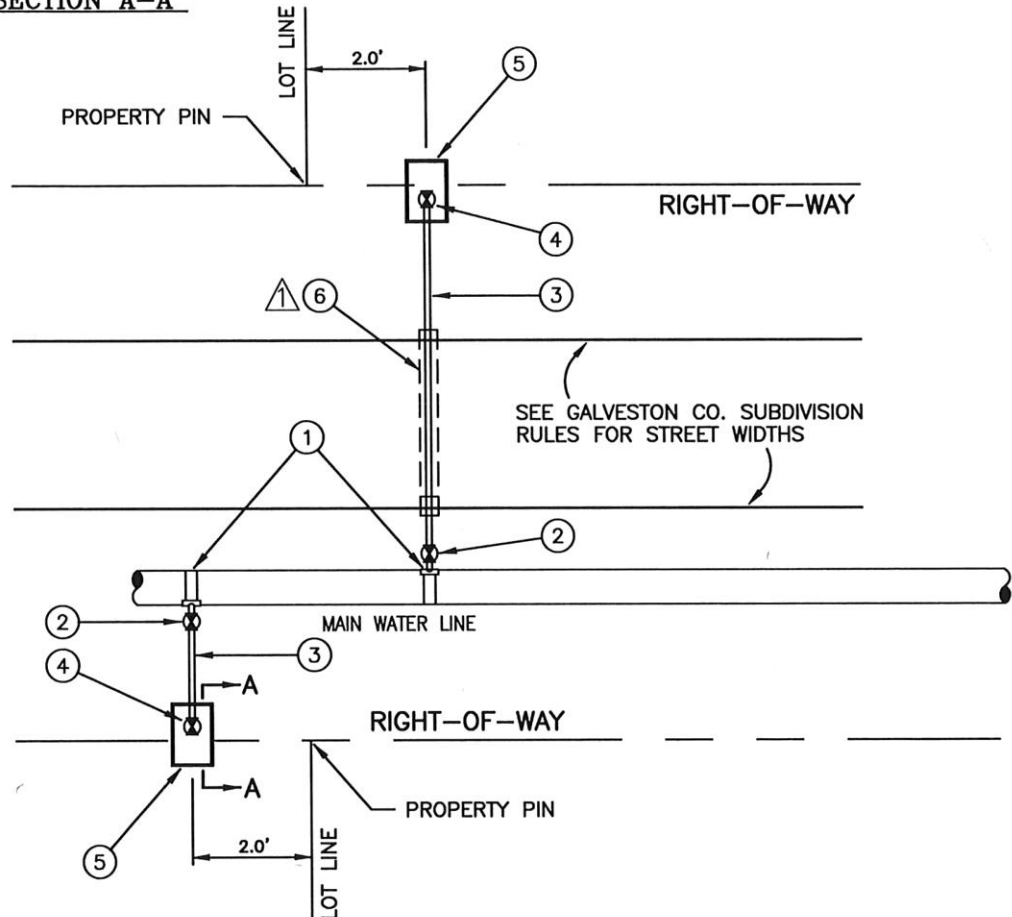
SECTION A-A
